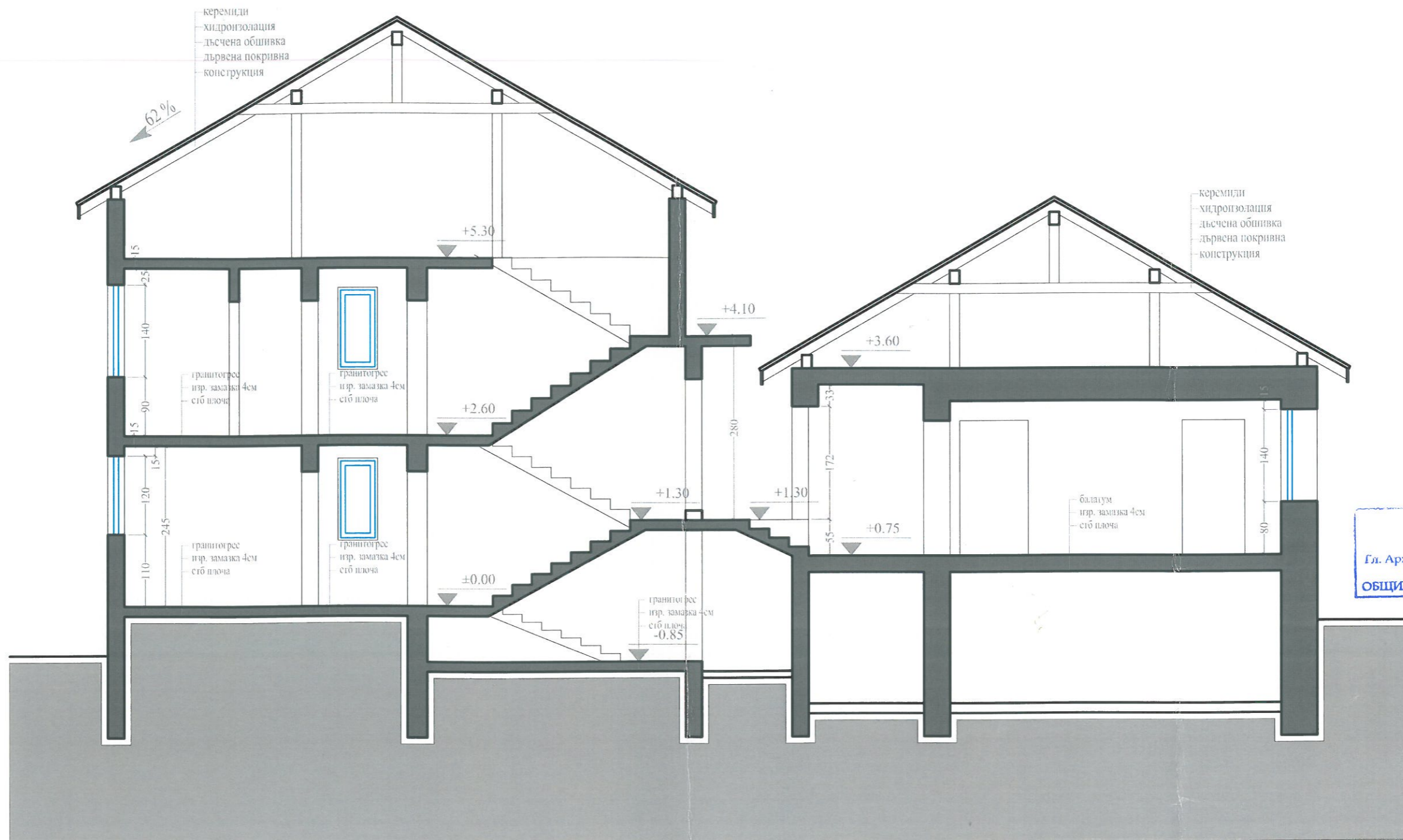
Разрез А - А
