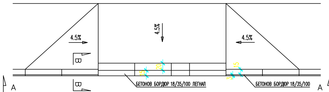
ИЗГЛЕД А-А М 1:50
