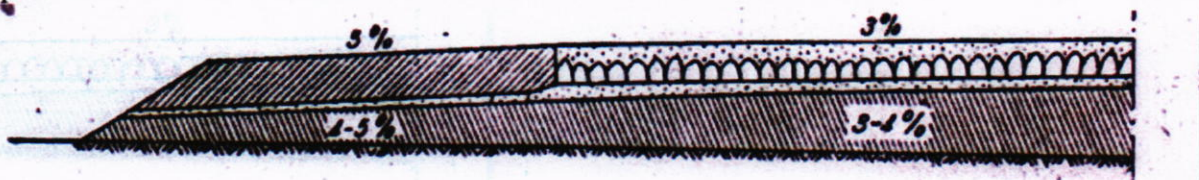
Фиг. 15. Напречен профил на трошенокаменна настилка с основен калдъръм и пясъчен слой
