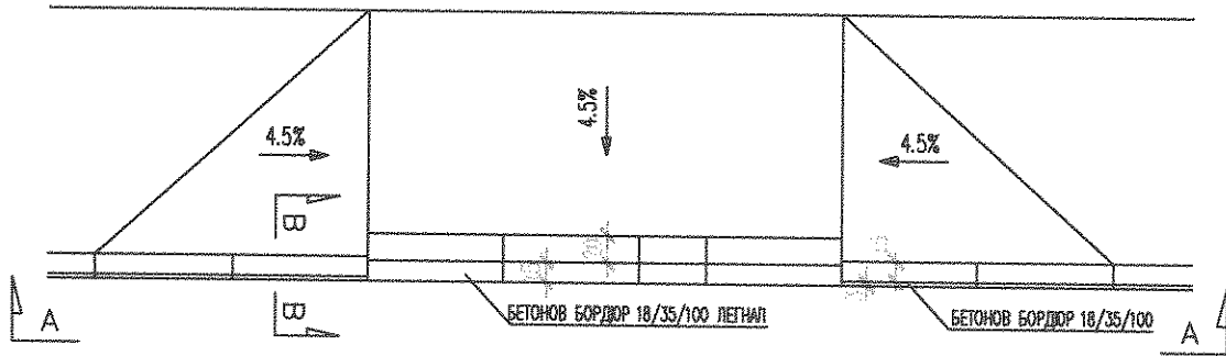
ИЗГЛЕД А-А М 1:50
