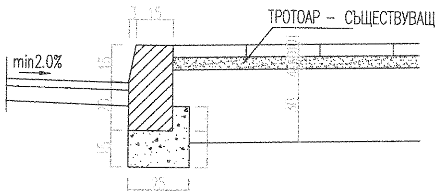
ДЕТАЙЛ "А3" М1:20 /БОРДЮР 18/35/
